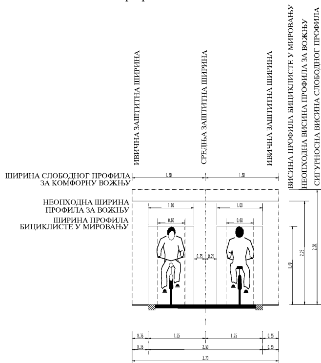
Слика 1 – Слободни профил бицикличке стазе
